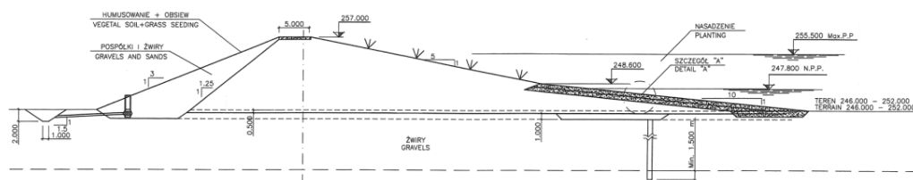
Fig. 4. Lateral dam Przyłek: cross-section in kms 0+000–3+600 according to [1]
