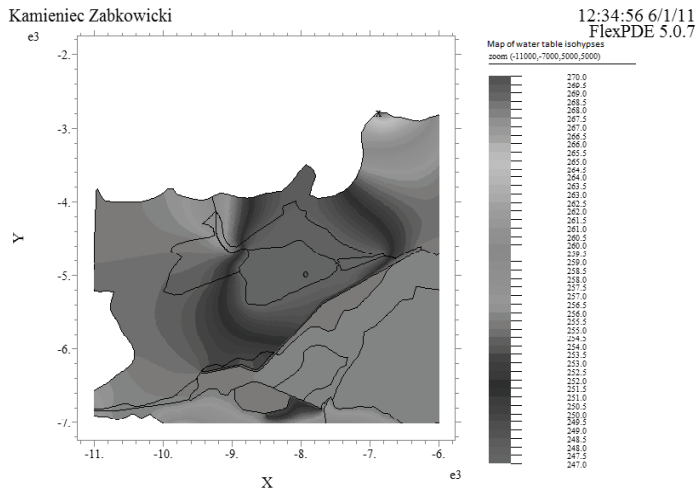
Fig. 11. Map of water table isohypses around Przylęk Polder
