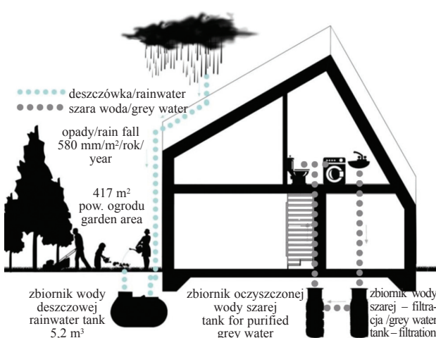
Il. 7. Schemat gospodarki wodnej – odzysku wody deszczowej oraz filtracji wody szarej (autor: A. Potaczek)
