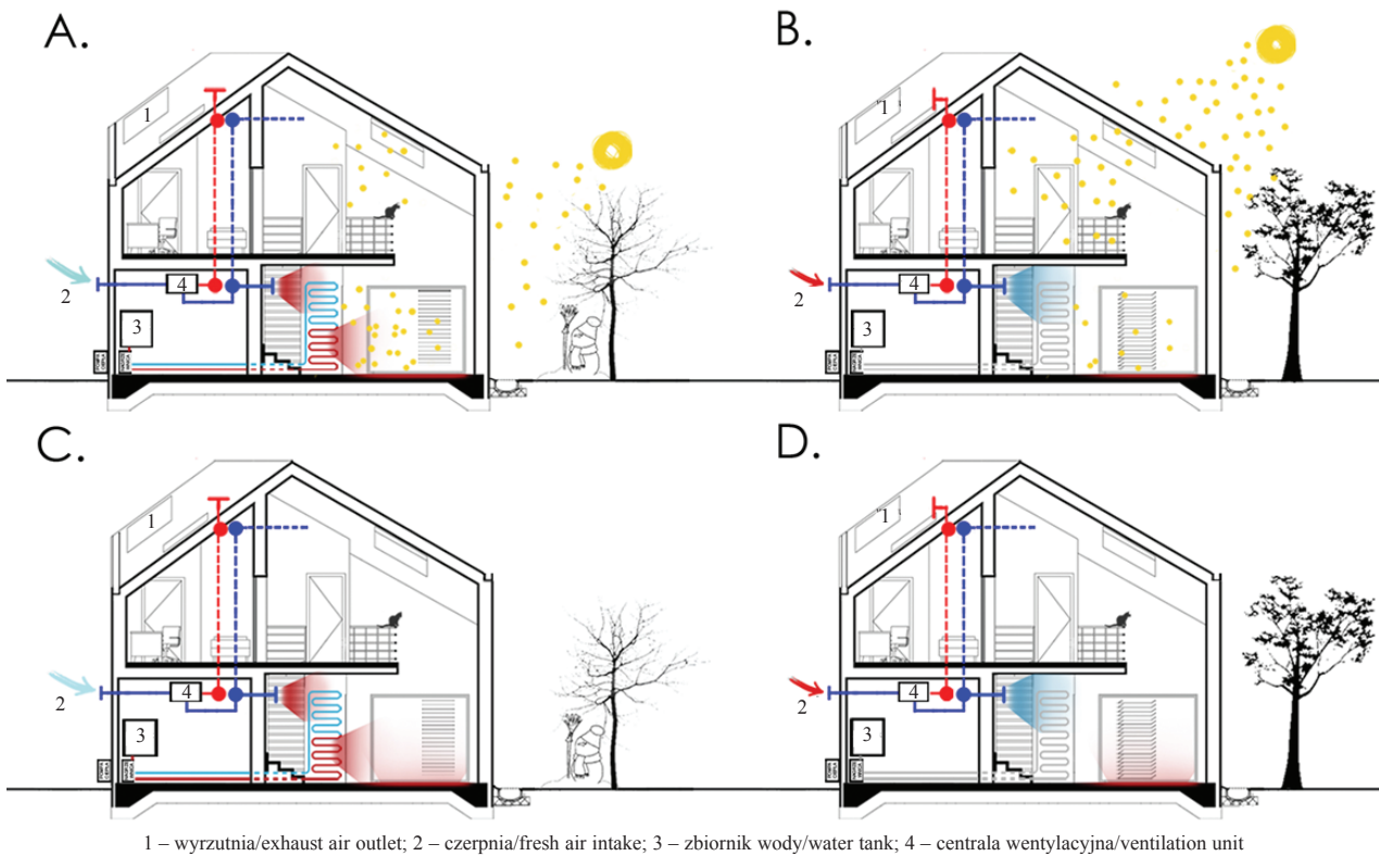
Il. 6. Schematy energetyczne dla projektowanego budynku o różnych porach dnia i roku. A – okres zimowy – dzień. Włączone jest ogrzewanie płaszczyznowe oraz wentylacja mechaniczna. Przesłony słoneczne na południowej elewacji ustawione są tak, aby przez przeszklenia wpadało do wnętrza jak najwięcej promieni słonecznych, ogrzewając powietrze oraz podłogę, która akumuluje ciepło. B – okres letni – dzień. Ogrzewanie płaszczyznowe jest wyłączone. Powietrze chłodzi wentylacja mechaniczna. W celu ochrony przed przegrzaniem przesłony słoneczne na południowej elewacji ustawione są tak, aby przez przeszklenia wpadała umiarkowana ilość promieni słonecznych. Podłoga, na którą padają promienie słoneczne, akumuluje ciepło. C – okres zimowy – noc. Włączone jest ogrzewanie płaszczyznowe oraz wentylacja mechaniczna. Dodatkowo ciepło emitowane jest przez podłogę, która akumuluje ciepło za dnia. D – okres letni – noc. Komfort temperatury zapewnia wentylacja mechaniczna, odpowiednio powietrze chłodząc lub ogrzewając. Ciepło akumulowane przez podłogę za dnia emitowane jest do wnętrza domu (autor: A. Grudzińska)
