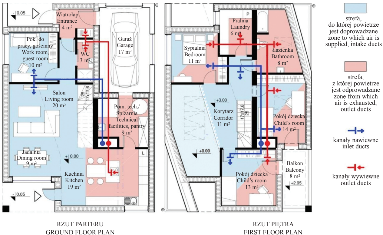
II. 4. Schematy instalacji wentylacji mechanicznej z odzyskiem ciepła w projektowanym budynku (autor: A. Grudzińska) Fig. 4. Installation plans of mechanical ventilation with heat recovery in the building (author: A. Grudzińska)
