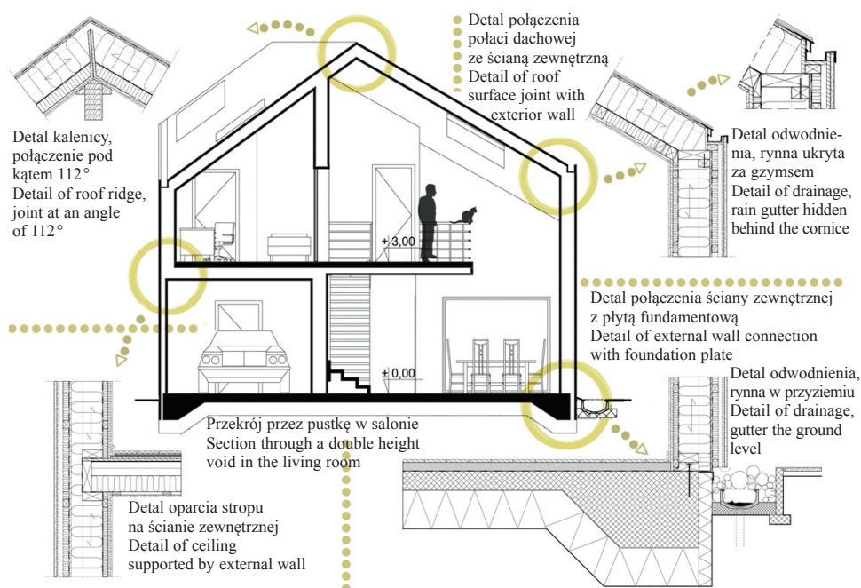
II. 3. Detale projektowe – rozwiązania połączeń przegród budowlanych w budynku. Lekki szkielet drewniany stanowią dwuteowe słupy oraz belki stropowe [3] (autor: A. Grudzińska) Fig. 3. Construction details – key junctions of building partitions. The lightweight wood frame construction consists of I-joint wall and ceiling studs [3] (author: A. Grudzińska)
