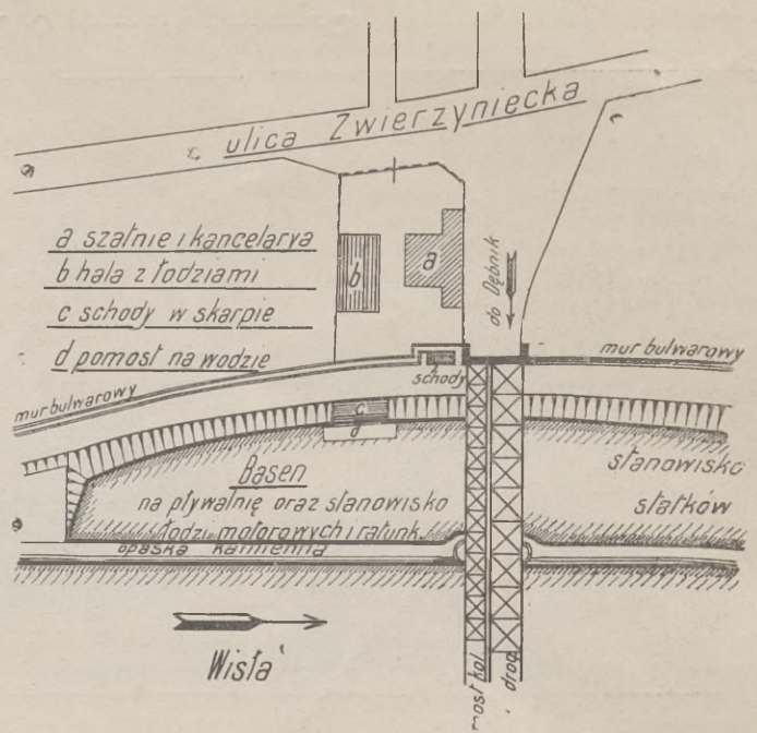
Plan sytuacyjny nowej przystani O. W. „Sokoła“ krak.
