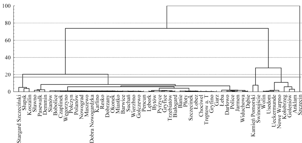
Rys. 1. Dendrogram Warda – miasta Pomorza Pruskiego według struktury rzemiosł
