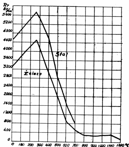
Rys. 2 Wykres spadku wytrzymałości stali i żelaza przy wzroście temperatury
