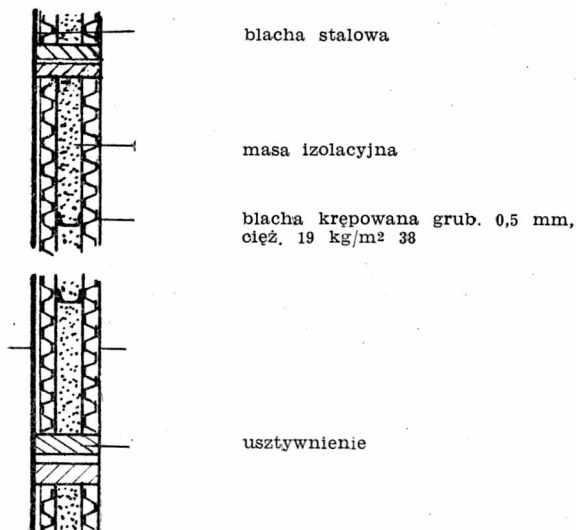
Rys. 4 Przekrój grodzi pożarowej typu niemieckiego
