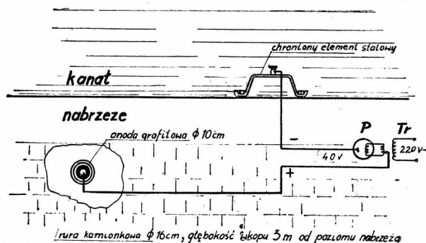
Rys. 6 Schemat instalacji ochrony katodowej z zewnętrznego źródła prądu w kanale portowym w Gdańsku (z anodą zakopaną w ziemi)
