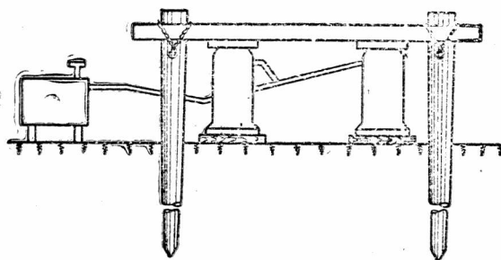
Wyciąganie pali za pomocą pras hydraulicznych
