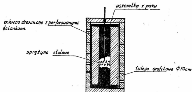
Rys. 5 Szczegóły umocowania anody grafitowej
