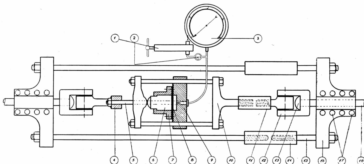
Dynamometr hydrauliczny-membranowy
