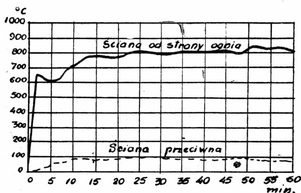
Rys. 3 Wykres temperatury po obu stronach grodzi pożarowej typu niemieckiego
