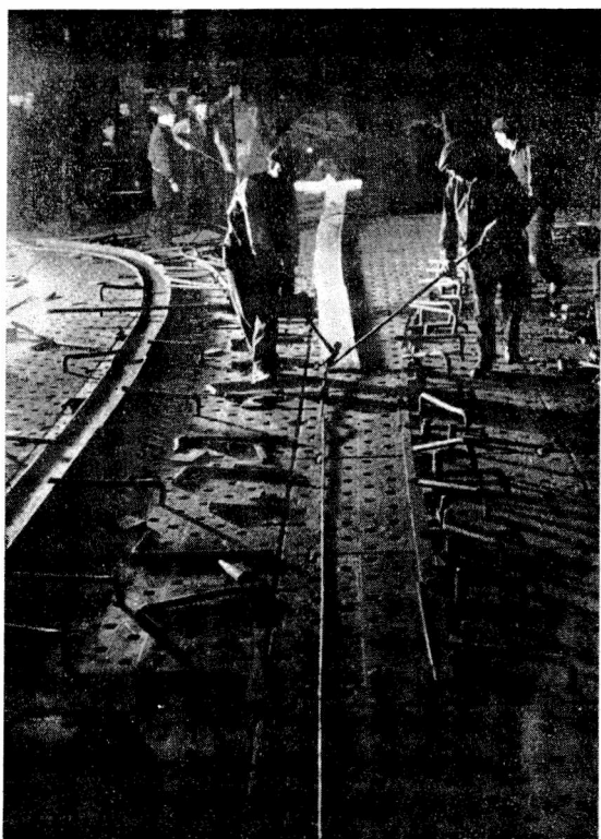
a) Początek operacji gięcia wręgu
