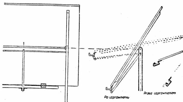
Rynienka na przybory do desek kreślarskich
