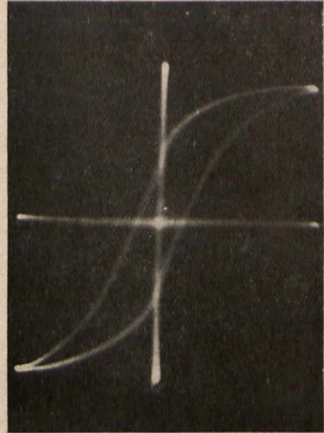
Rys. 17. Krzywa histerezy dla próbki z zelaza lanego — f = 50 okr/sek.
