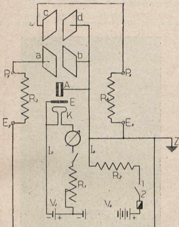
Rys. 12. Układ połączeń oscylografu Western Electric Co
