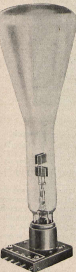
Rys. 13. Widok rury z żarzoną katodą.
