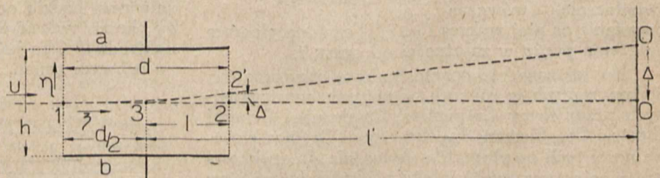
Rys. 4. Odchylenie elektronów przez pole elektryczne.
