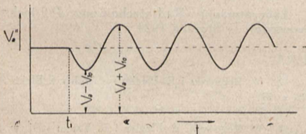
Rys. 28. Napięcie o częstotliwości badanej włączone w obwód anodowy rury.
