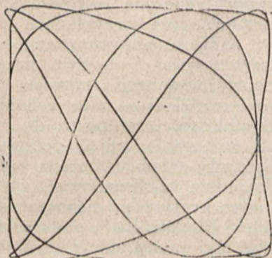
Rys. 27. Krzywa Lissajou dla stosunku częstotliwości 4:5
