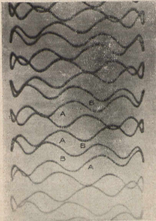
Rys. 9. Oscylacje niezankające o częstotliwości 2 160 000 okr/sek (w/g Dufour'a).
