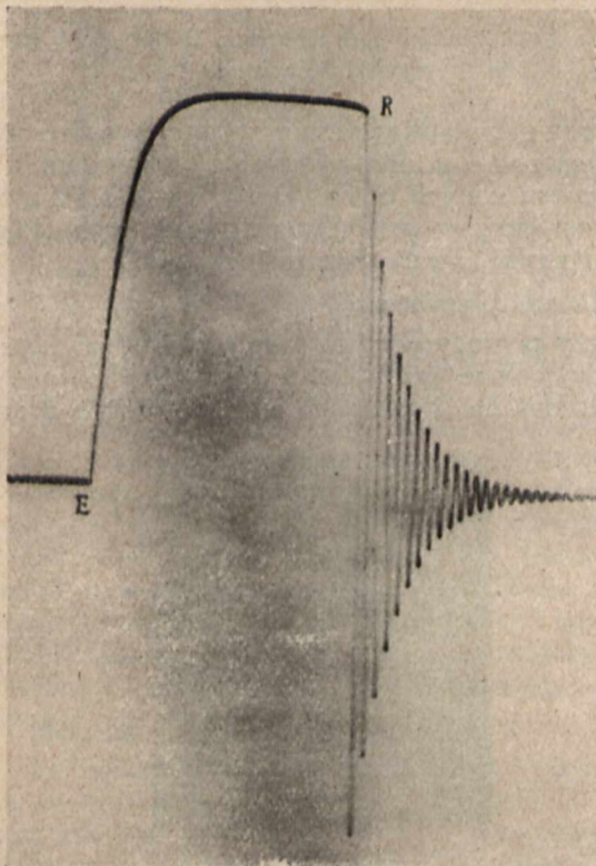
Rys. 5. Załączenie i przerwanie prądu stałego w obwodzie z cewką indukcyjną bez rdzenia — równoległe do przerywacza włączony kondensator (w/g Dufour'a).
