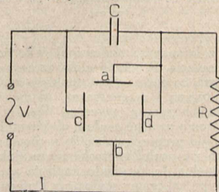
Rys. 14. Obwód z pojemnością C i oporem R .
