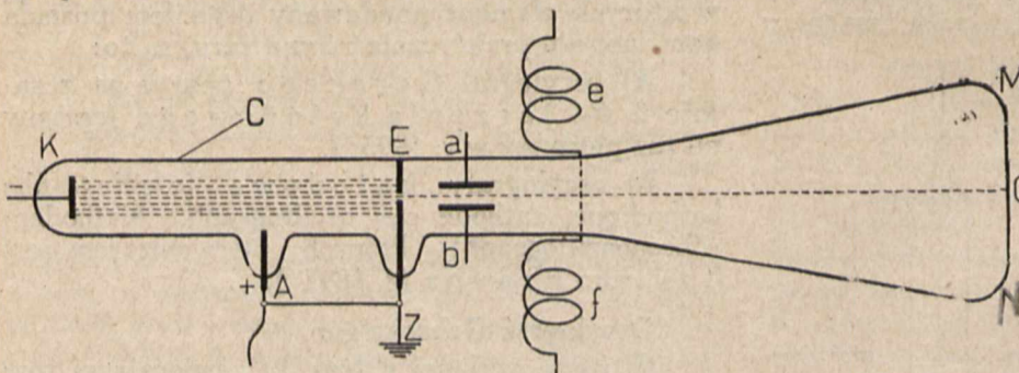
Rys. 3. Schemat rury Brauna'a.
