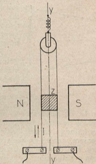
Rys. 1. Schemat oscylografu pętlicowego.
