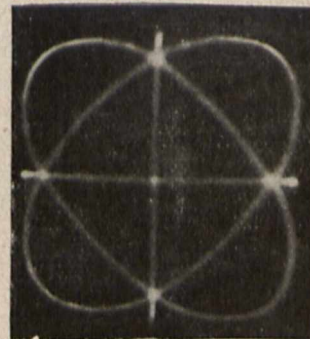
Rys. 11. Krzywe Lissajou dla 2 napięć przesuniętych w fazie o 60° i 120°.
