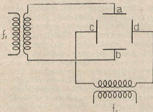
Rys. 24. Układ do porównywania częstotliwości.
