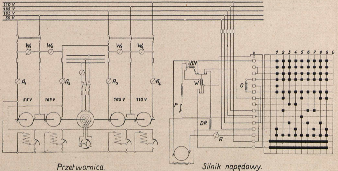
Rys. 17. Układ połączeń dla napędu drukarek przy systemie pięcioprzewodowym.
