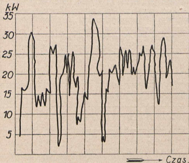
Rys. 4. Obciążenie silnika przy napędzie grupowym 4-ch przedzarek okresowych.
