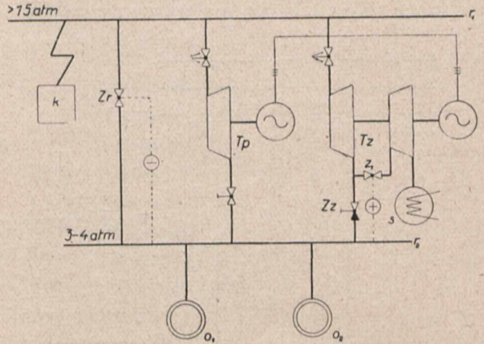
Rys. 21. Elektrownia fabryczna przy zapotrzebowaniu energii elektrycznej, przewyższającym zapotrzebowanie pary. K — kocioł z przegrzewaczem, Zr — zawór redukcyjny, Tp — Turbina przeciwprężna, Z2 —zawór zwrotny, Z1 — rozrząd części niskoprężnej, S — skraplacz, v1 i v2 — rurociągi parowe, o1 i o2 — odbiorniki pary.
