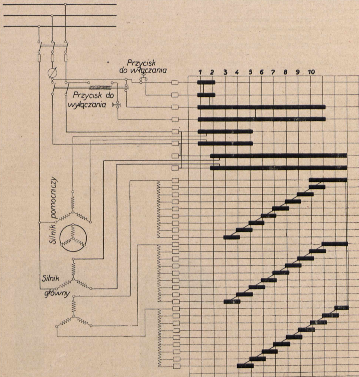
Rys. 19. Układ połączeń przy napięciu dwusilnikowym wykładziarki.
