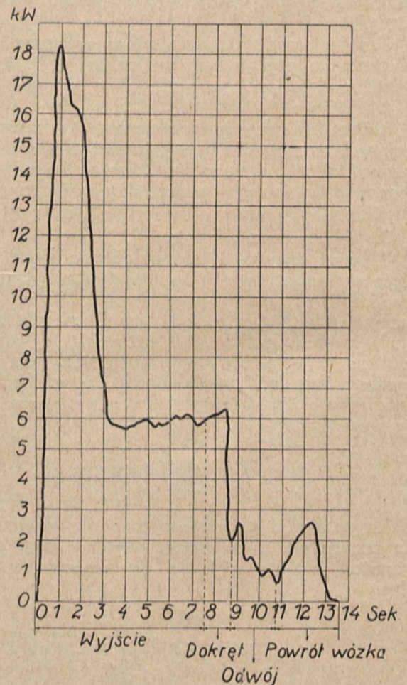
Rys. 2. Praca przędzarki okresowej o 600 wrzecionach. i 7500 obrotów wrzeciona.
