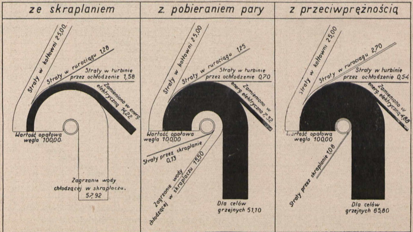
Rys. 20. Porównanie bilansów cieplnych turbogeneratora o mocy 1000 kW przy pracy.
