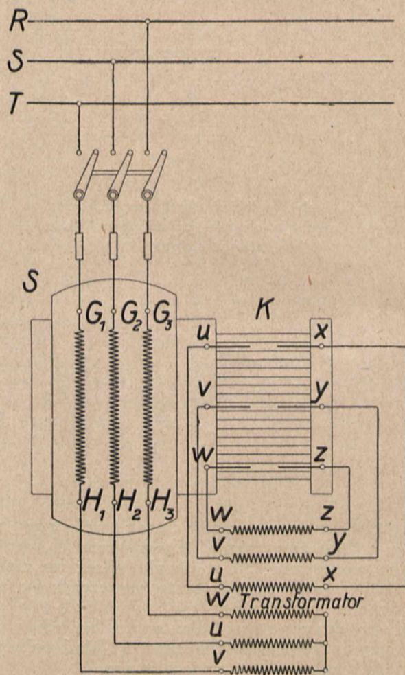
Rys. 7. Układ połączeń silnika kolektorowego trójfazowego szeregowego.
