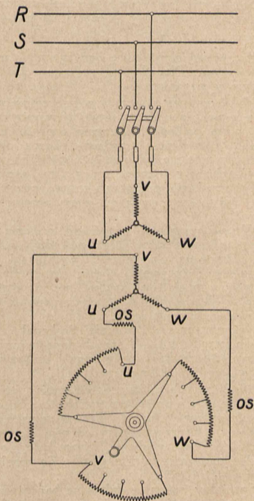
Rys. 3. Układ połączeń silnika asynchronicznego z oporami stałymi w obwodzie wirnika.
