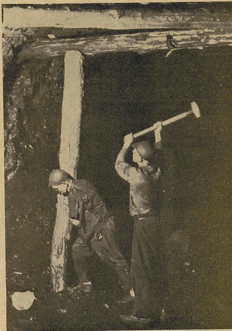
Podbijanie stempli w kopalni węgla.
