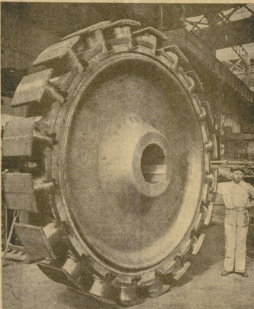
Biegunowe koło magnetyczne z lanej uszlachetnionej stali.
