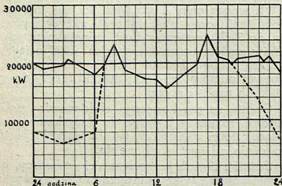
Rys. 1-d. Doba największego obciążenia.
