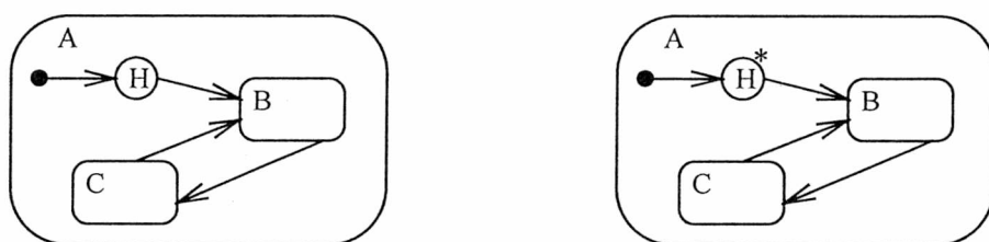
Rys. 2.7 Przykład zaznaczania płytkiej i głębokiej historii
