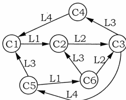
Rys. 5.3 Zredukowany diagram Łącucha Markowa
