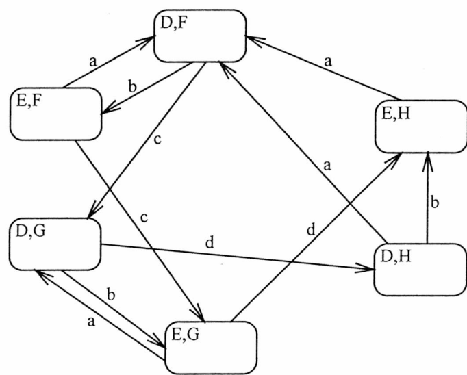
Rys. 2.6b Płaska specyfikacja systemu z rys. 2.6a
