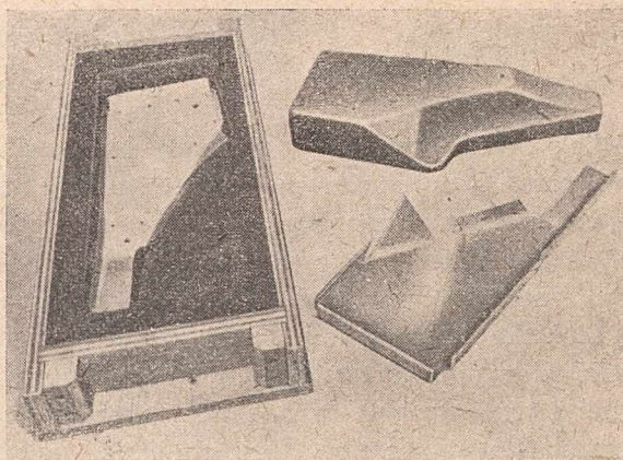
Forma do tłoczenia o skomplikowanych kształtach.
