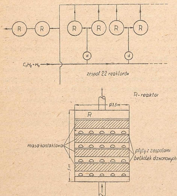
Rys 2 Katalityczne uwodornienie acetyleny
