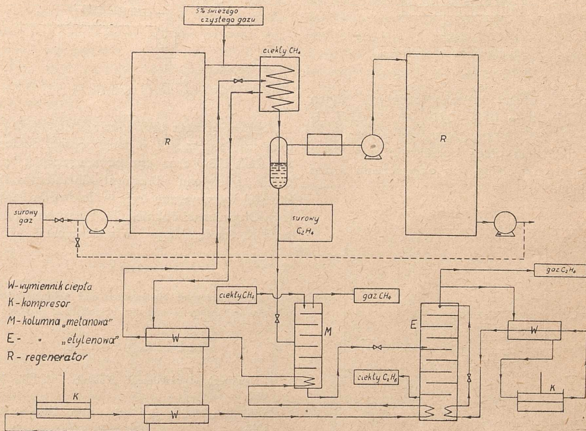
Rys 1 Otrzymywanie etylenu z gazu koksowniczego
