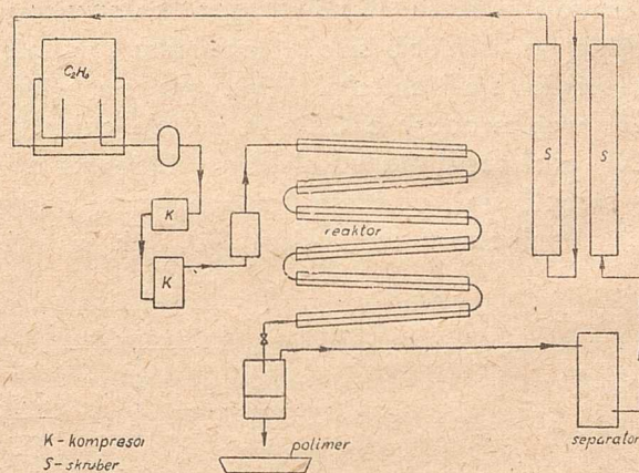
Rys 4 Schemat syntezy LUPOLEN-u H
