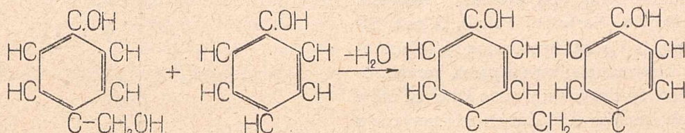
p-dwuhydroksydwufenylometan
