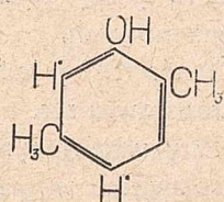
2,3-ksylenol
