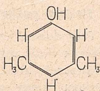
3,5-ksylenol
