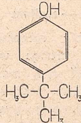
butylofenol
