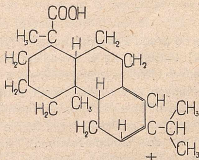
kwas abietynowy.
