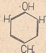
p-krezol
