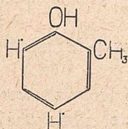
o-krezol
