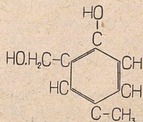
o-metylo-o-p-krezol
