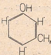
m-krezol
