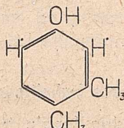
3,4-ksylenol
