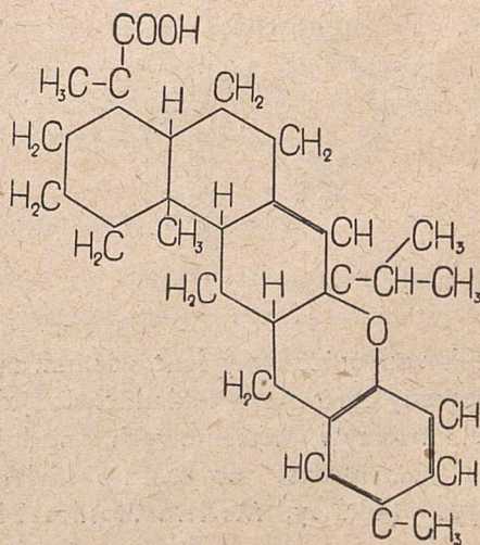
kwas albertolowy
