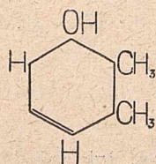
2,5-ksylenol
