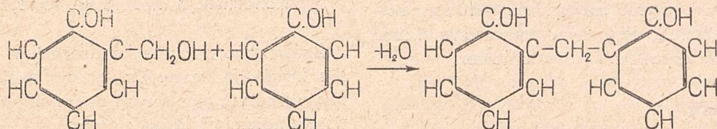
o-dwuoksydwufenylometan
