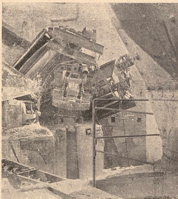
Dwa młyny pierścieniowe w fabryce superfosfatu
