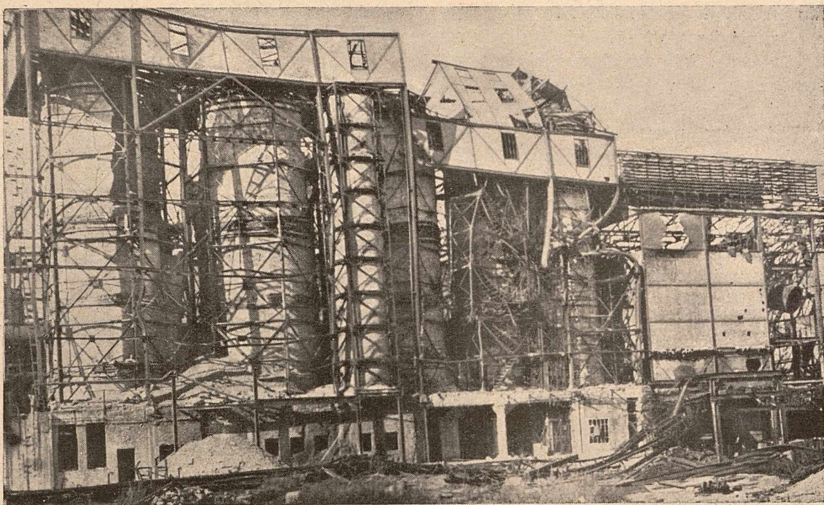
Instalacja do produkcji kwasu siarkowego metodą wieżową w fabryce superfosfatu
