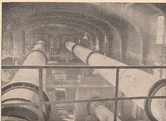
Widok na halę pieców obrotowych
