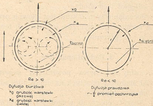
Rys. 1. Graficzne przedstawienie dwu charakterystycznych wypadków dyfuzji
