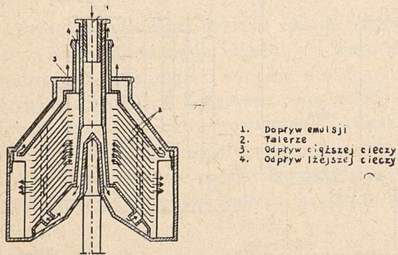
Rys. 3. Przekrój przez tętn wirówki
