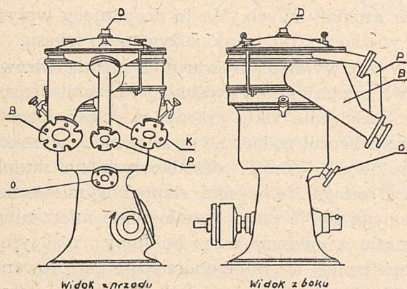
Rys. 2. Wirówka kwasowa
