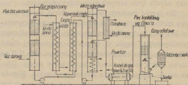
Schemat urządzenia do usuwania siarki z gazu met. alkacidowa i G
