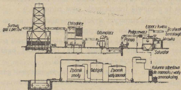
Schemat aparatury met. półpośredniej usunięcia amoniaku z gazu wg Koppersa
