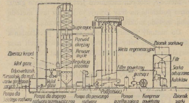
Schemat aparatury wg metody Thylox Koppers Co
