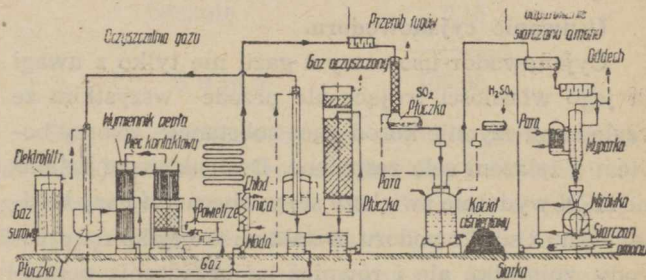
Schemat aparatury metody Katasulf
