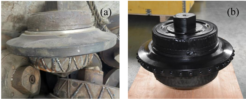
Fig. 1. The disc hob: (a) CS hob, (b) ST hob
