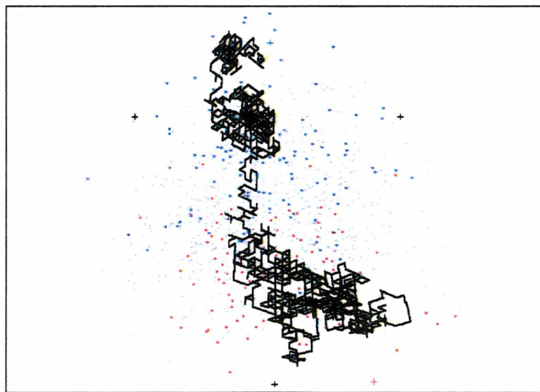
Rysunek 9.6: Trajektoria poszukiwań algorytmu SA.
