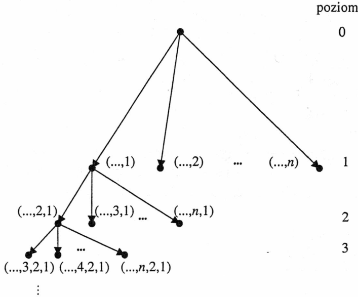
Rysunek 8.1: Drzewo \mathcal{H} .
