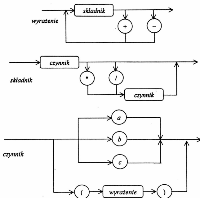
Rys. 5.2. Diagramy składniowe gramatyki G_W
