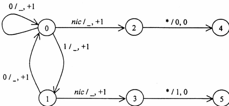
Rys. 4.5. Diagram przejść pomiędzy stanami
