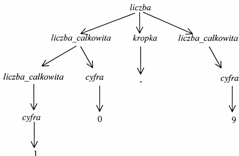
Rys. 5.1. Drzewo wywodu słowa 10.9
