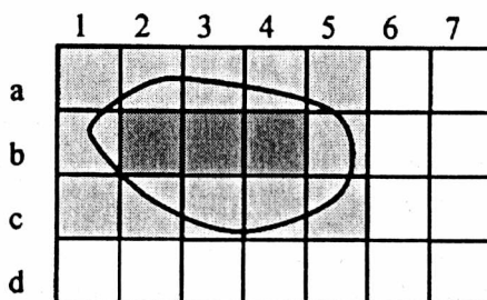
Rys. 4.2. Graficzna ilustracja zbioru przybliżonego
