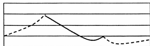
Rys. 4.1. Graficzna ilustracja operacji na zbiorach rozmytych
