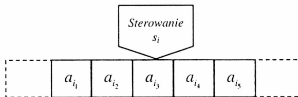
Rys. 4.3. Maszyna Turinga
