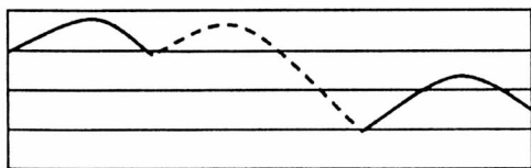
Funkcja przynależności sumy dwóch zbiorów rozmytych
