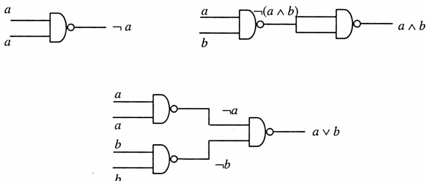
Rys. 7.3. Przykładowe schematy układów logicznych
