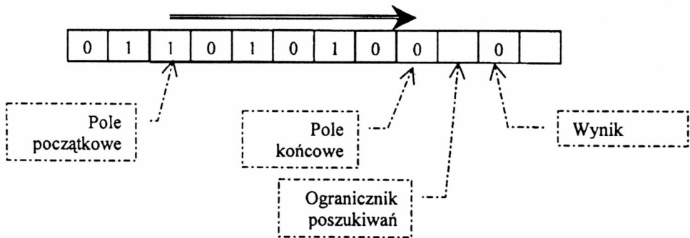
Rys. 4.4. Przykładowa zawartość taśmy
