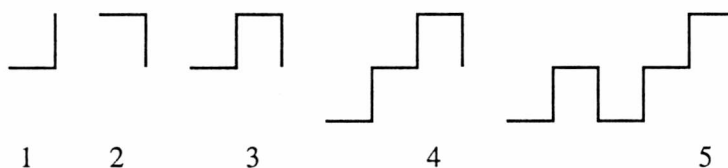
Rys. 2.1. Elementy zbioru LinieŁamane
