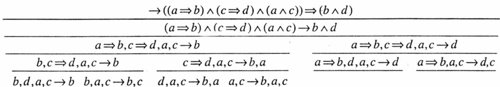
Rys. 9.1. Drzewo dowodowe dla formuły (1)
