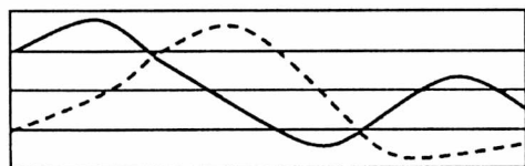
Funkcje przynależności dwóch zbiorów rozmytych – linia ciągła i linia przerywana
