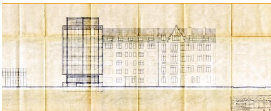
Fasada budynku Polikliniki Politechniki Wrocławskiej przy ul. Janiszewskiego. Projekt: Leszek Zdek, 1973 r.
