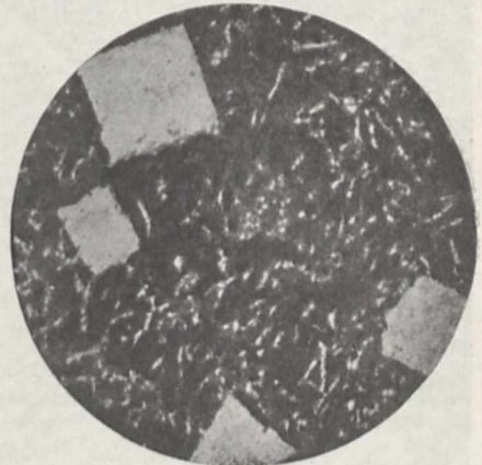
FIG. 2.—Alloy of tin, 90 per cent.; antimony, 10 per cent.
