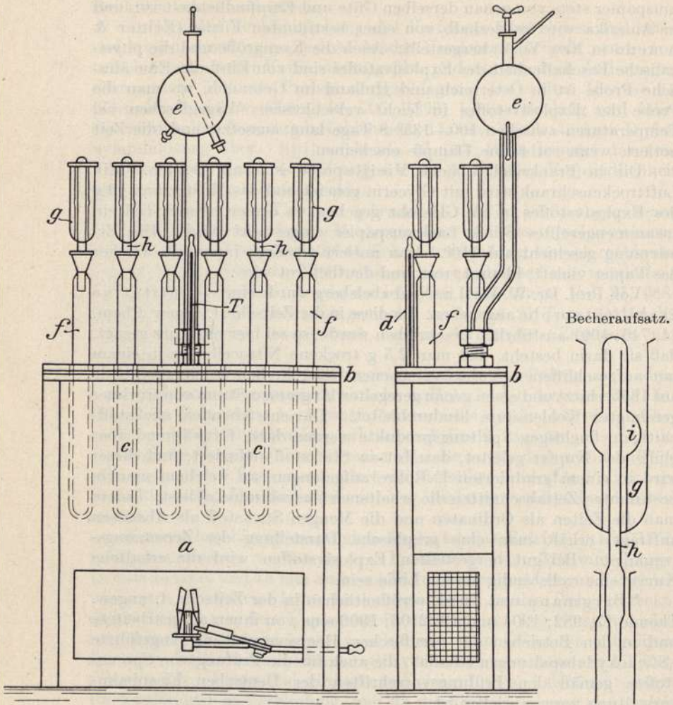
Vorderansicht.
