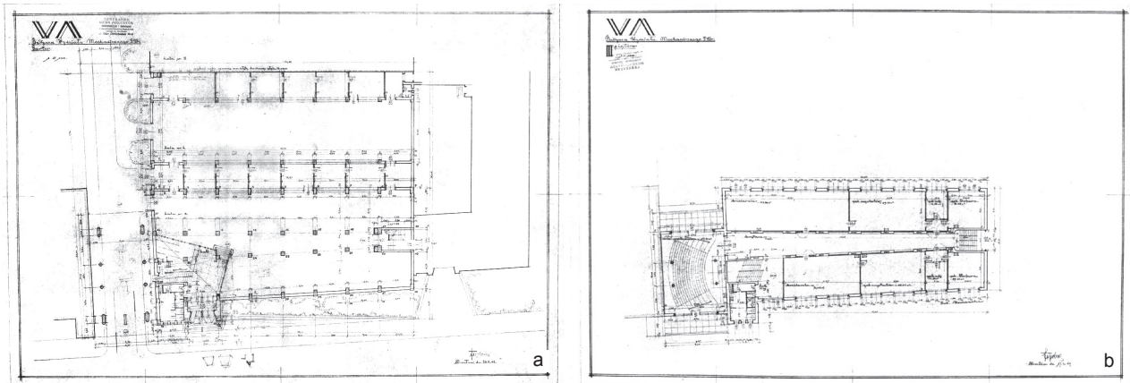
Il. 3. Wrocław, ul. Łukasiewicza, gmach główny Wydziału Mechanicznego, rzuty: a) parteru, b) III piętra (proj. A. Frydecki, 1949) (Muzeum Architektury we Wrocławiu, sygn.: MAt IIIc-P/59P/4, MAt IIIc-P/54/3)
