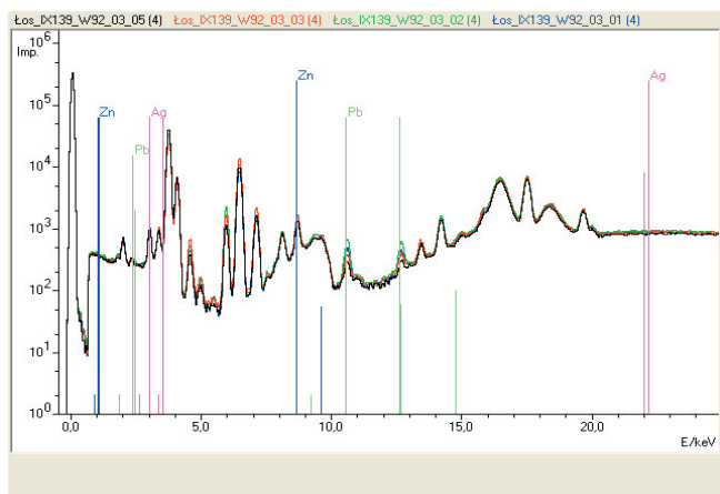
Ryc. 7. Wyniki XRF z jakościowej analizy żarna nr inw. 139_w. 92; podwyższona zawartość Pb, Ag i Zn; najwyższe stężenie ołowiu w punkcie 02 (zielona linia)
