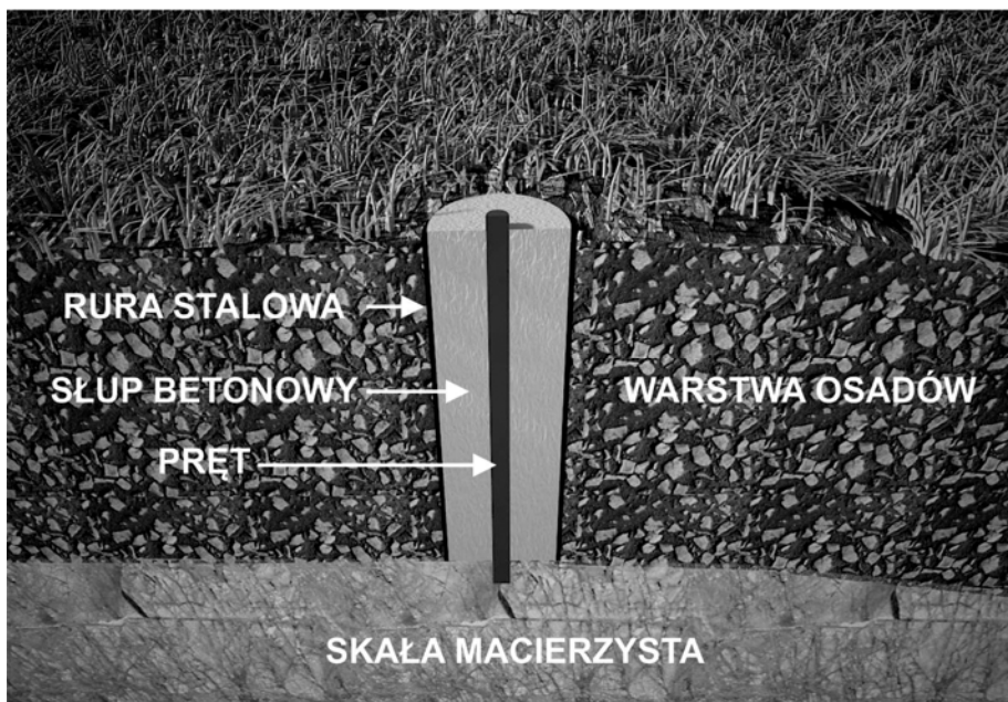
Rys. 3. Widok sposobu stabilizacji punktów geodezyjnych (opracowanie własne)
