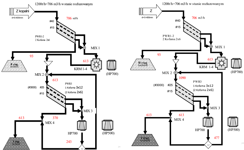
Rys. 1. Podstawowy układ technologiczny poddany analizie i ocenie. Przez wyłączenie lub zmianę elementów otrzymujemy struktury (tab.1). W nawiasach alternatywne maszyny i/lub ich parametry.
