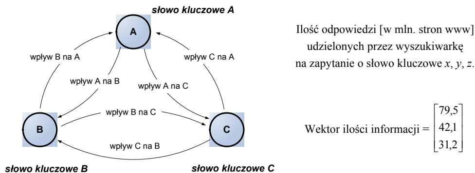
Rys. 2. Graf i wektor informacji dla trzech słów kluczowych x, y, z .
