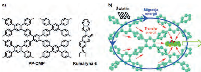
Rysunek 8. a) struktura PP-CMP oraz kumaryny 6; b) schematyczna reprezentacja obiegu energii z PP-CMP do przestrzennie ograniczonej kumaryny 6. Umieszczono za zgodą z [17]. Prawa autorskie 2010, Journal of the American Chemical Society
