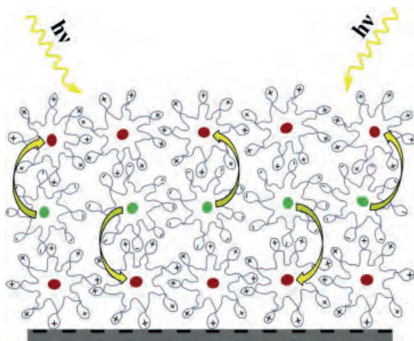
Rysunek 5. Schematyczna ilustracja micelarnej wielowarstwy zbudowanej z amfilowych polielektrolitów z chromoforami osadzonymi w hydrofobowych micelach. Zaznaczone zostały fotoindukowane procesy transferu energii/elektronu pomiędzy odizolowanymi molekułami donora (zielone kółka) i akceptora (czerwone kółka) przebywającymi w sąsiednich warstwach. Umieszczono za zgodą z [21]. Prawa autorskie 2015, European Polymer Journal
