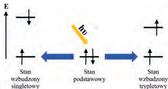
Rysunek 1. Absorpcja światła prowadzi do przeniesienia elektronu ze stanu podstawowego do stanu wzbudzonego: singletowego (lewa strona) lub trypletowego (prawa strona)
