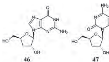
Rysunek 2.3. Struktura 3'-deoksyguanozyny i 3'-deoksycytydyny
