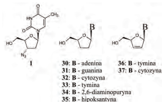
Rysunek 1.1. Niektóre 2',3'-dideoksynukleozydy
