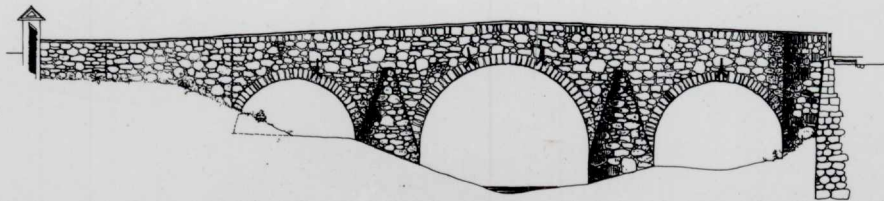
ANSICHT
