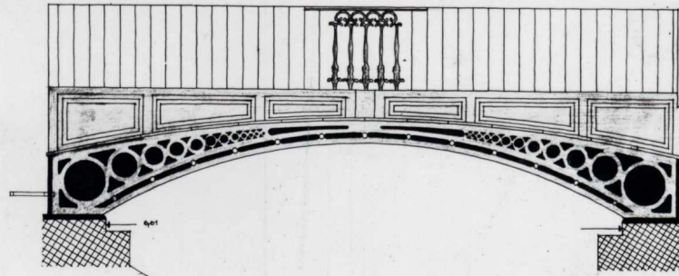
ANSICHT
