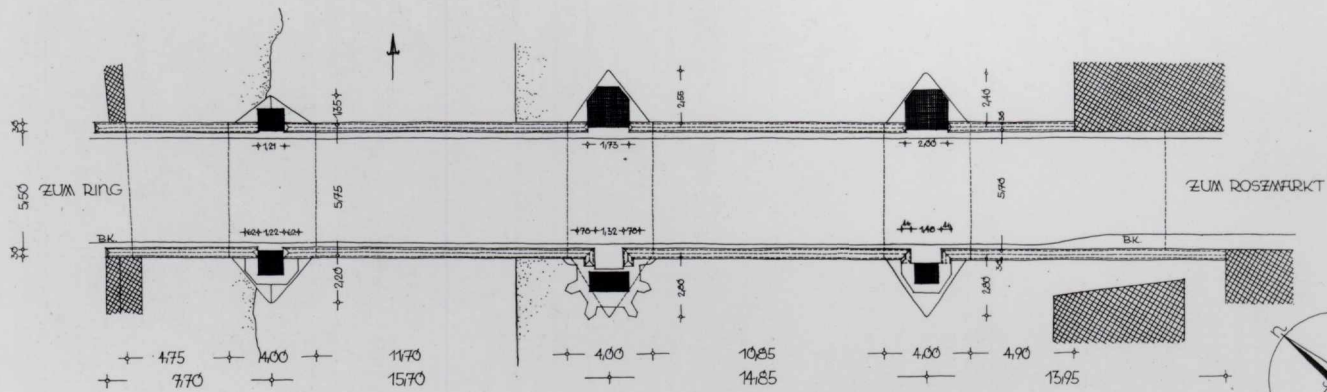
GRUNDRIß
