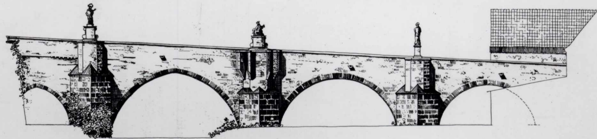
SÜDANSICHT
