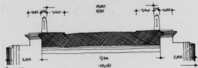
SCHNITT
