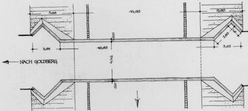
ANSICHT UND DRAUFSICHT + M.// 1:100.
