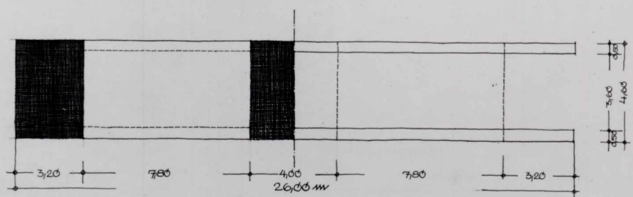
DRAUFSICHT UND SCHNITT.
