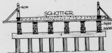
ANSICHT UND SCHNITTE M // 1:50.
