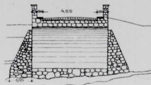
SCHNITT
