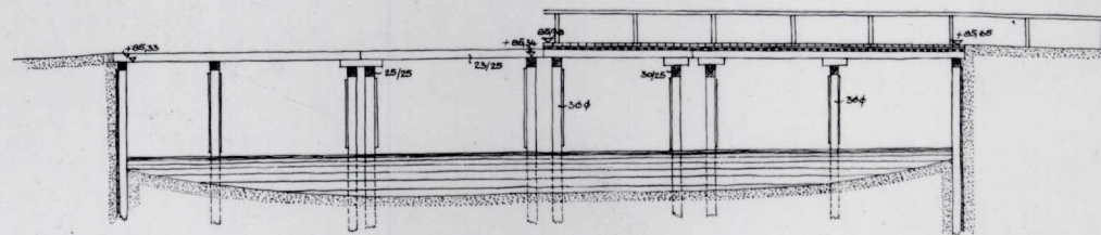
SCHNITT UND ANSICHT M/1:100.
