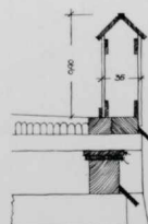
PUNKT E M/1:20 ALLES ANDERE M/1:100.
