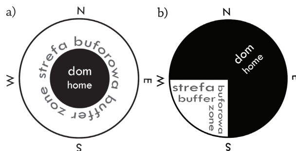
Il. 2. Schematy funkcjonalne budynków ze strefami buforowymi: a) strefa buforowa wokół pomieszczeń ogrzewanych, b) strefa buforowa wbudowana pomiędzy pomieszczenia ogrzewane (oprac. W. Lechowska)
