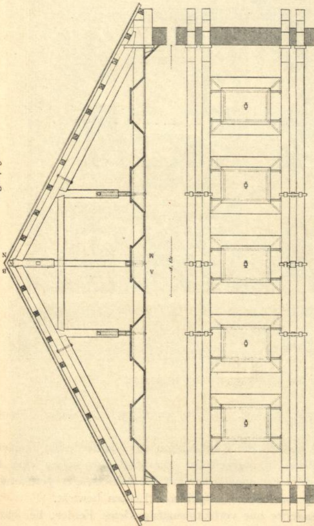
Deckenkonstruktion in der Kirche Santa Maria maggiore zu Rom 1140 w. Gr.
