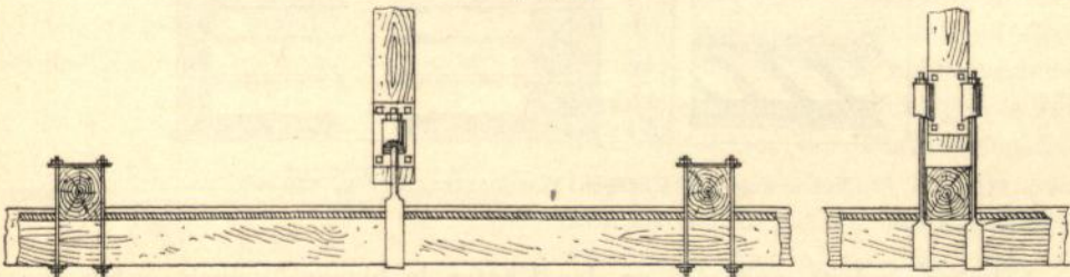
Deckenkonstruktion mit Oberstützen und angehangener Balkenlage.
