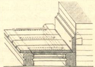
Amerikanifcher kalfatertes Fußboden 43) .
