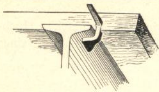
Rordorf's Verbindungshafte.
