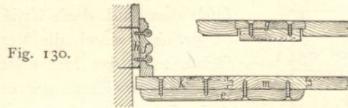
Befestigung des Fußbodens an eisernen Trägern (D. R.-P. Nr. 11 141 51) ).
