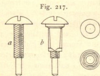
Teppichschrauben. w. Gr.
