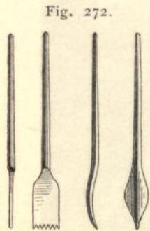
Werkzeuge für Ausführung des Sgraffito 139) .
