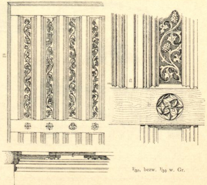
Gestülpt verschalt Balkendecke 218) .
