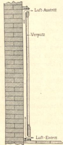
Falzbautafeln von Fischer . ca. \frac{1}{105} w. Gr.
