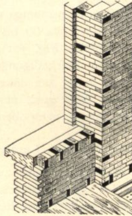
Vermauern von Katz'schen Dübelsteinen.
