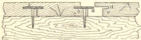
Fußboden mit eisernen Federn 39) . 1/15 w. Gr.
