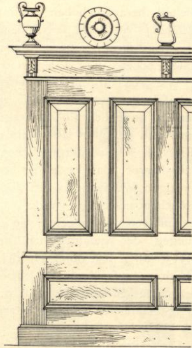
Wandbekleidung mit gestemtem Sockel und Gesims. \frac{1}{15} w. Gr.
