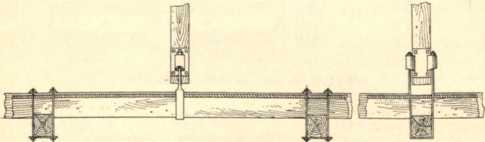
Deckenkonstruktion mit Unterstützen und aufgekämmter Balkenlage.
