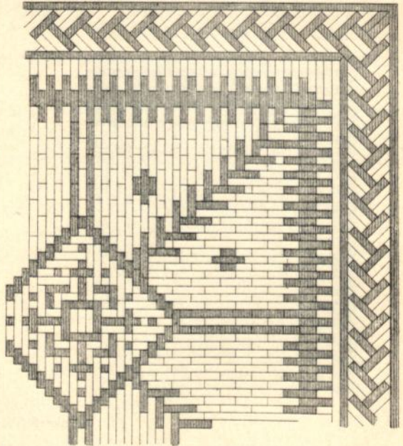
Klinkerfußböden 5) .
