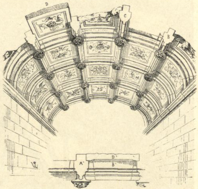
Kassettiertes Tonnengewölbe 184) .
