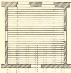
Dieling mit verfetzten Stößen. 1/200 w. Gr.
