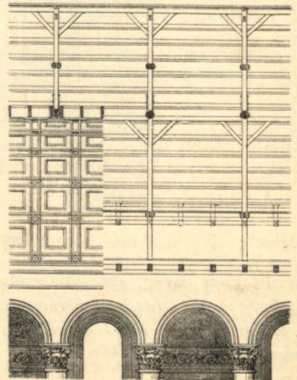
Längenschnitt zu Fig. 472 225) .
