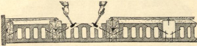
Deckenbildung nach dem System Efch.
