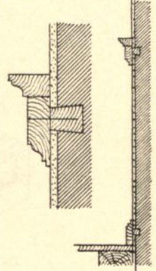
Wandleiste.
