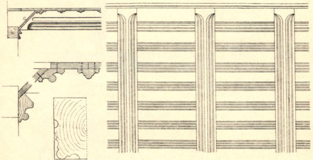
Balkendecke mit befäumten Fußbodenbrettern 211) .
