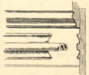
Verzierte gestülpte Bretter 211 ).
