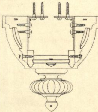
Hydrolitdecke.
