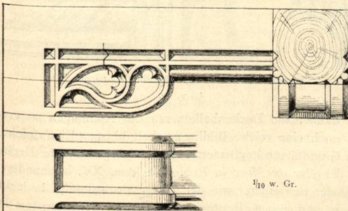
Unterstützung des Deckenbalkens durch ein Sattelholz 205 ).
