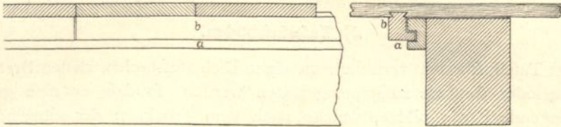
Tafelfußboden von Badmeyer 52) .
