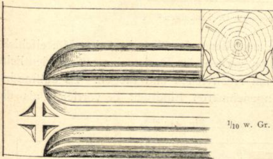
Balkenkehlungen 205 ).
