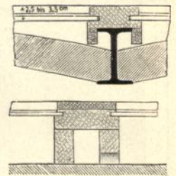
Hetzer'scher Fußboden über Gewölben 58 ).
