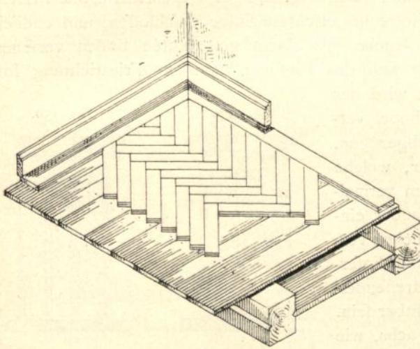
Riemchenfußboden.
