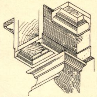
Umkleidung der Balken mit Brettern 217) .
