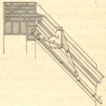
Ausführung geputzter massiver Gefimse 239) .
