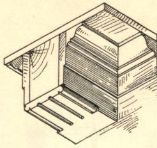
Umkleidung der Balken mit Brettern 217) .
