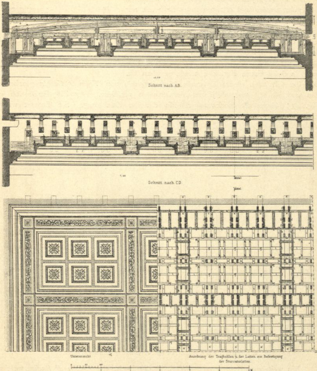
Befestigung der Kassetendecke an der Balkenlage 225 ).
