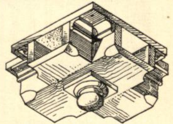
Gliederung der Decke durch hohle Kästen 217) .
