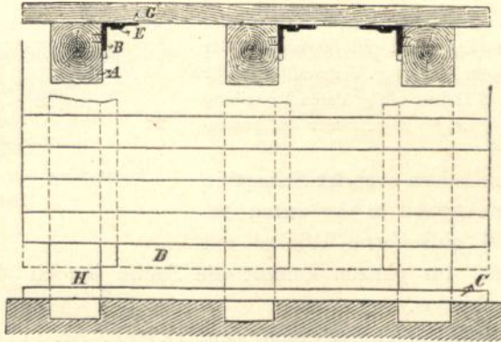
Fußboden mit verschiebbaren Brettern 48) .
