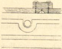
Dichtung der Fugen durch oberhalb der Einschubdecke aufgenagelte Leisten 211 ).
