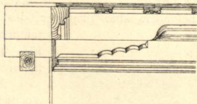
Unter 45 Grad gelegte Einschubdecke 211 ), \frac{1}{10} w. Gr.
