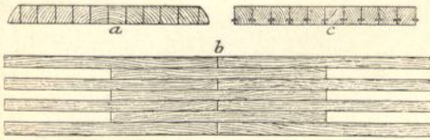
Holzplatten-Fußboden von Schultze 54 ).
