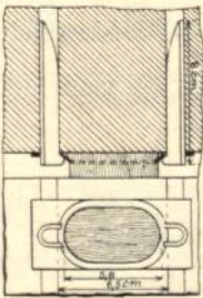
Mauerdübel von Thicke .
