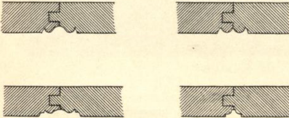
An den Kanten profilierte Bretter.
