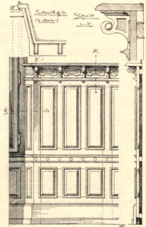
Anschluß der Wandbekleidung an das Fenster 156) .
