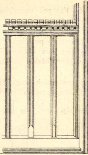
Wandbekleidung mit besäumten Brettern und Deckleisten 151) .
