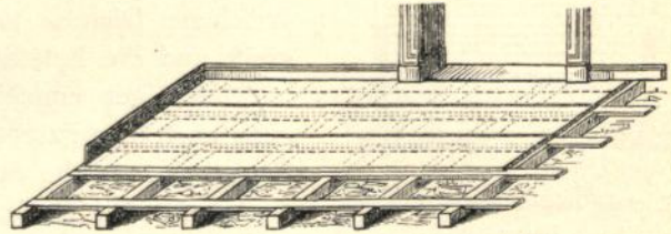
Sächfischer ungefpundeter Fußboden 43) .
