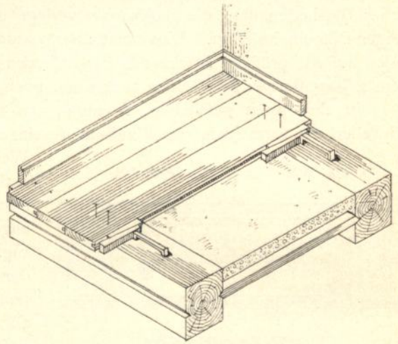
Verlegen des Fußbodens.
