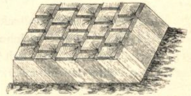
Klotzpflaster 71) .
