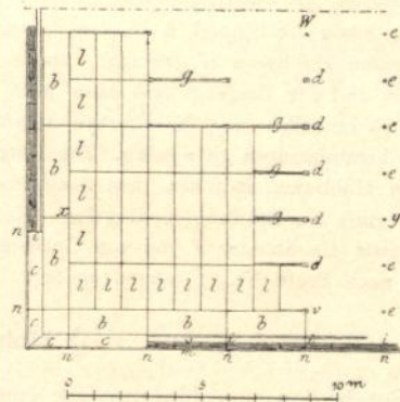
Übersichts-Grundriss des Fussbodens.
