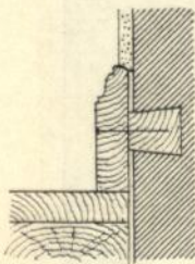
Fufsleifte mit anstossendem Wandputz.
