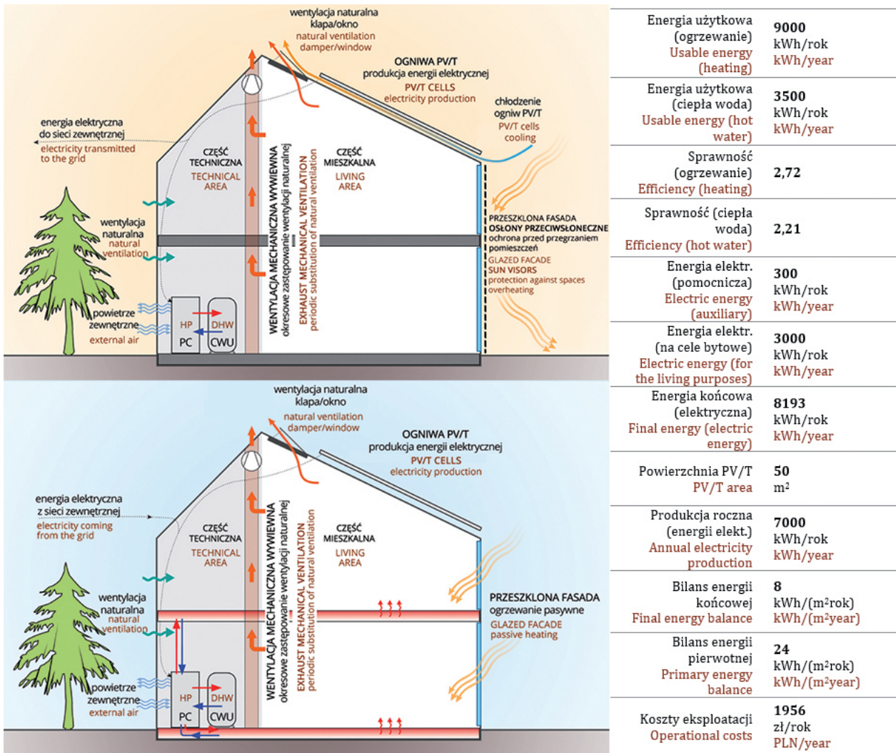
II. 1. Roczny bilans energii i kosztów eksploatacji w domu naturalnym; praca systemu w lecie (górny schemat) i w zimie (dolny schemat)
