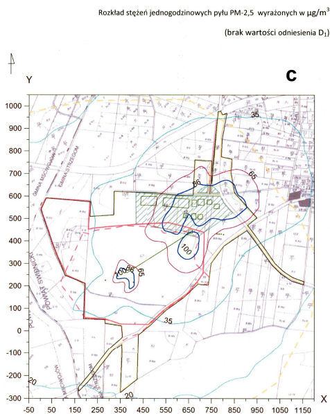
Rysunek. Rozkład stężeń a – \text{SO}_2 b – \text{NO}_2 c – \text{PM}_{2.5} d – \text{PM}_{10} , Figure. Distribution of concentration of: a – \text{SO}_2 b – \text{NO}_2 c – \text{PM}_{2.5} d – \text{PM}_{10}
